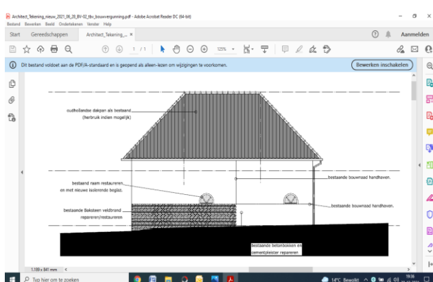
Voorgevel nieuw
